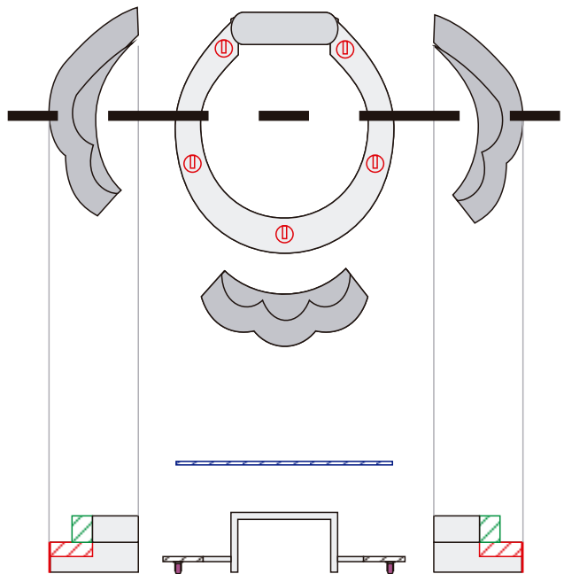
VISTA FRONTAL - DESPIECE CORTE
