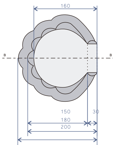
VISTA LATERAL - CERRADA
