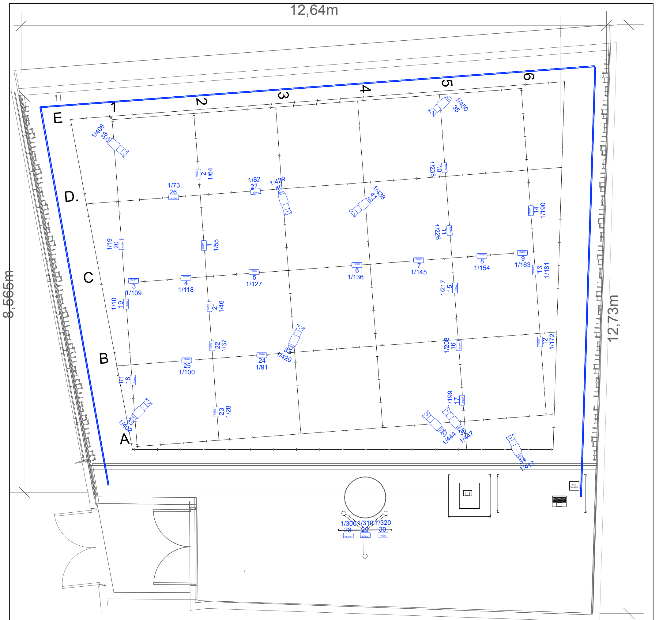
PLANTA Scale: 1:50
