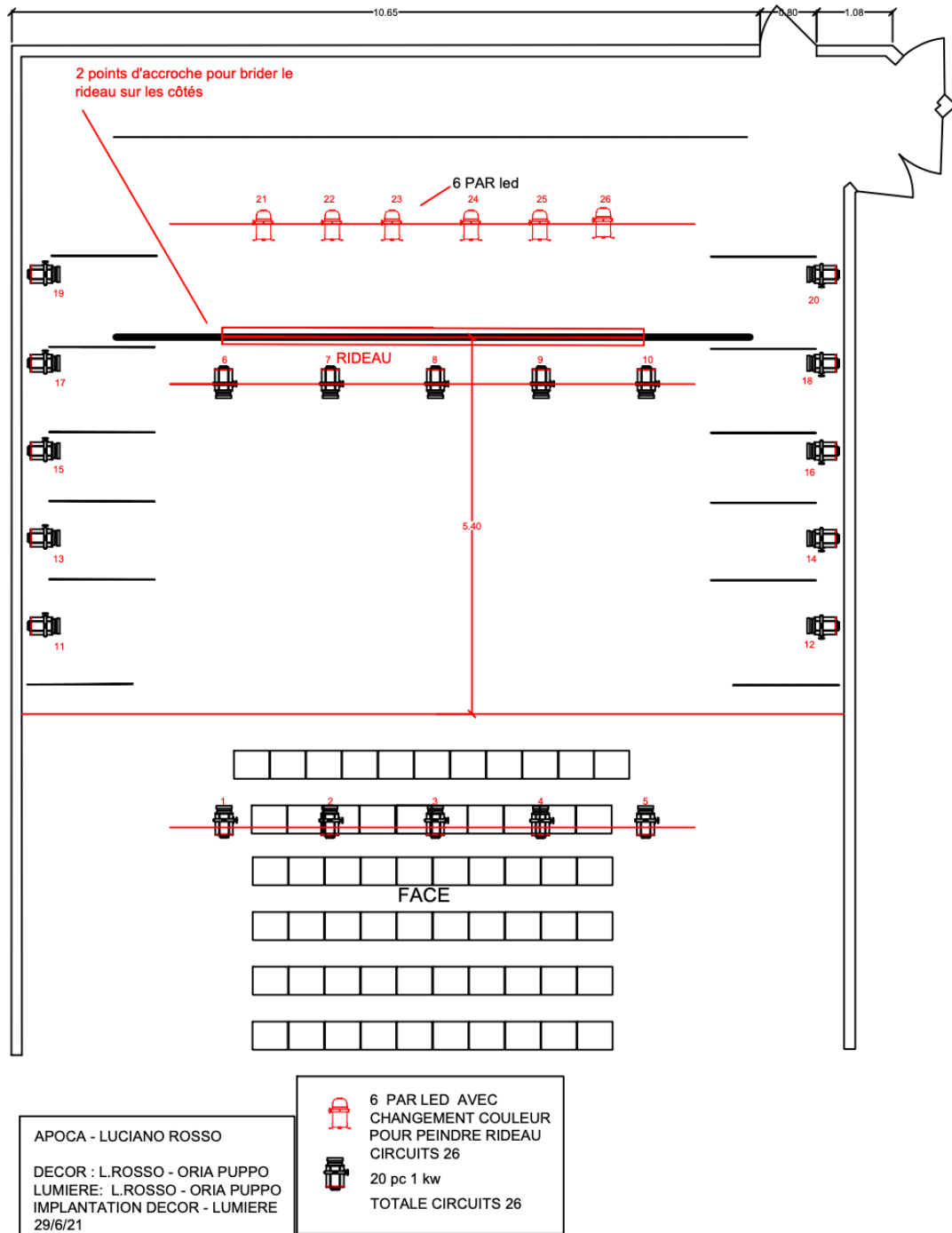
FIGURA 2 - PLANO DE LUCES
